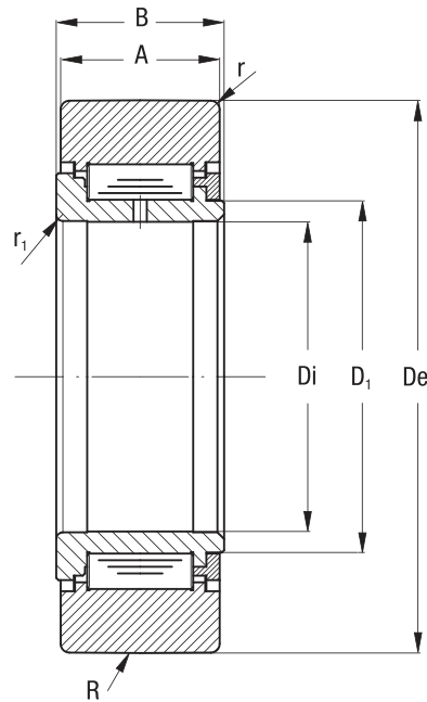
FGU 无密封圈 FGU ... MM金属密封圈
